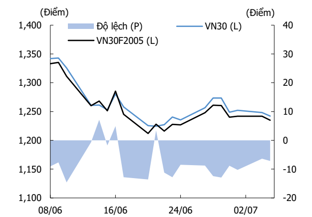
Hình 2. Basis spread
